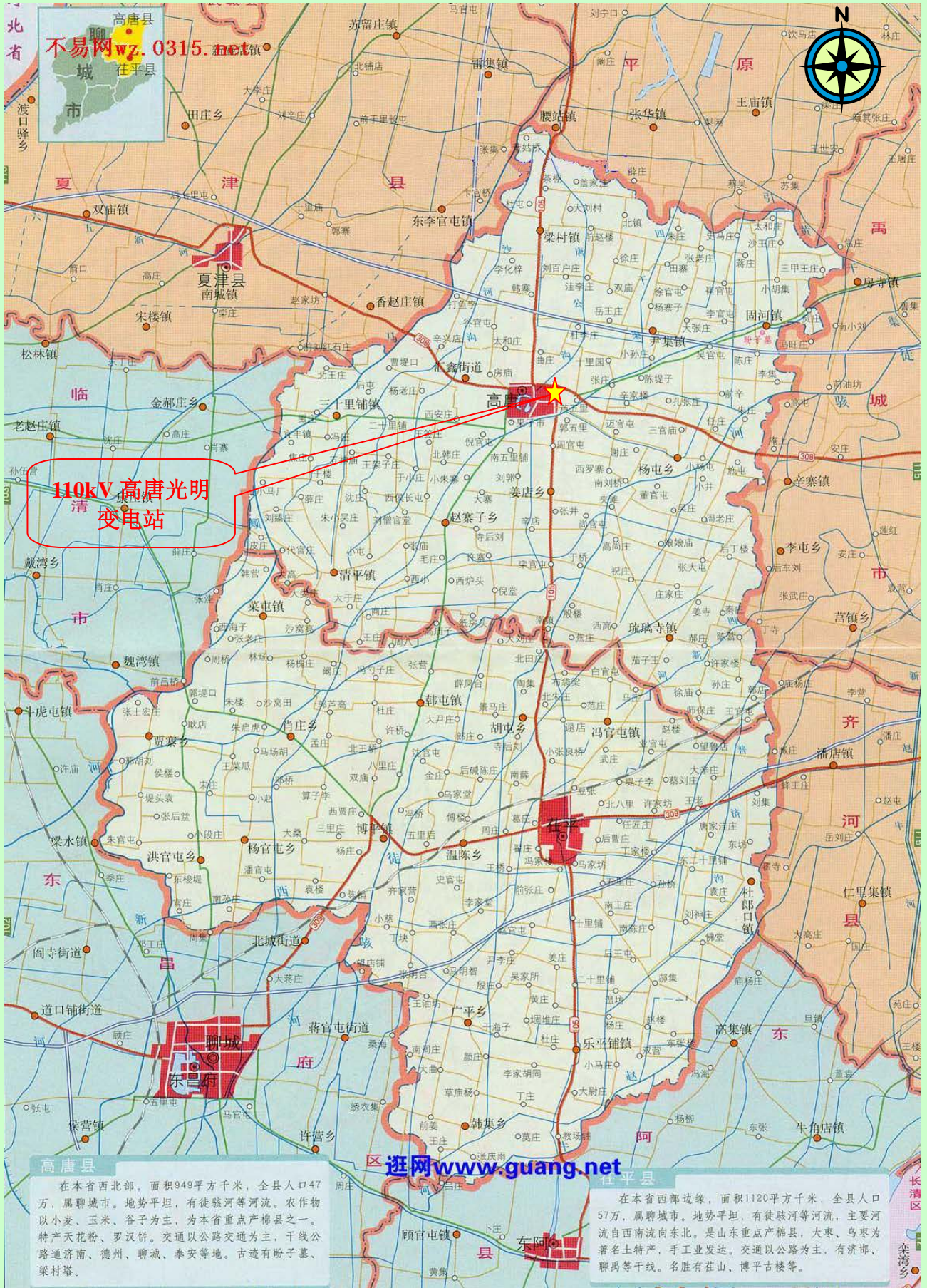
附图1 110kV 高唐光明站址区域位置示意图
