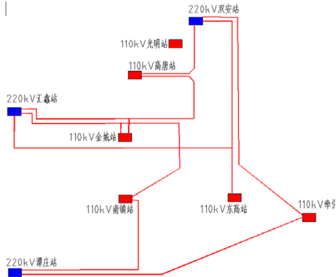
图 1 本工程电网改接前接线简图
