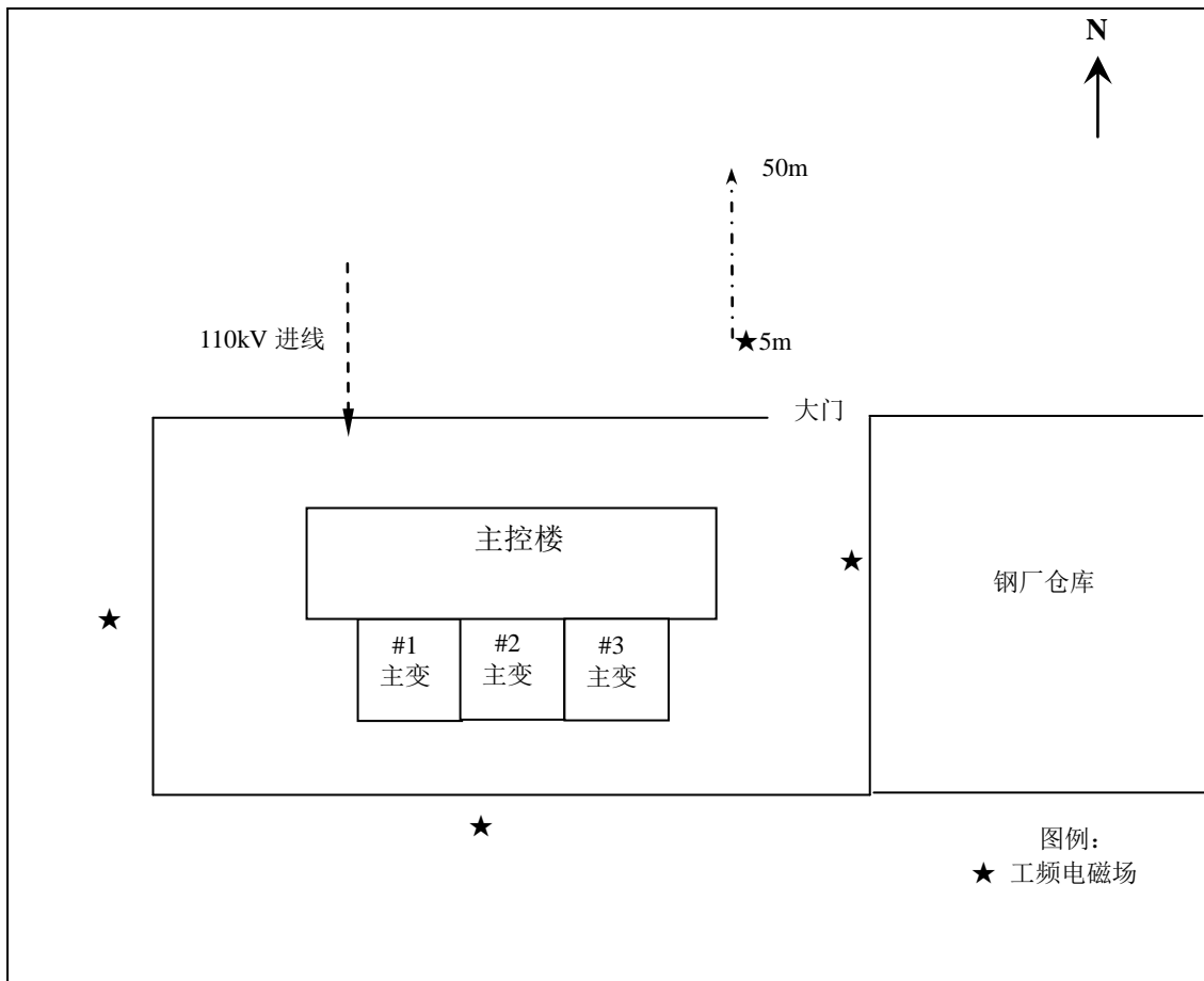
图 5 110kV 荣光变电站监测布点示意图
