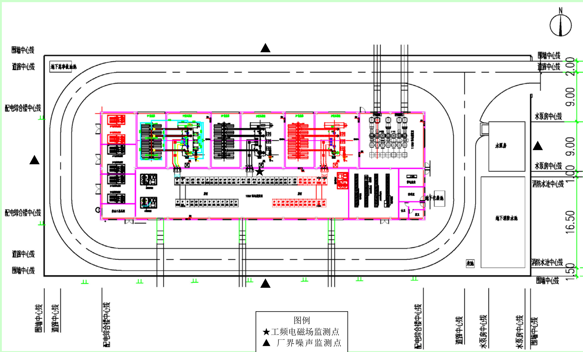
附图3 高唐光明站总平面布置及监测布点示意图
