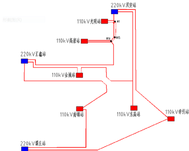
图 2 本工程电网改接后接线简图
