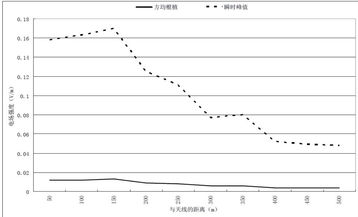
图 5-5 电场强度变化趋势图
