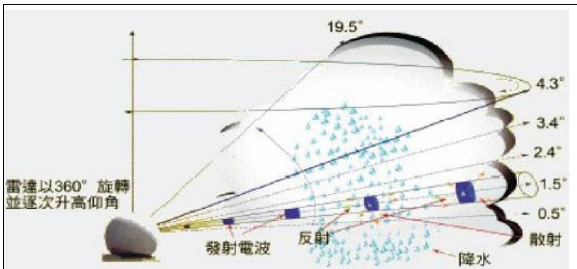
图 2-4 雷达探测示意图
