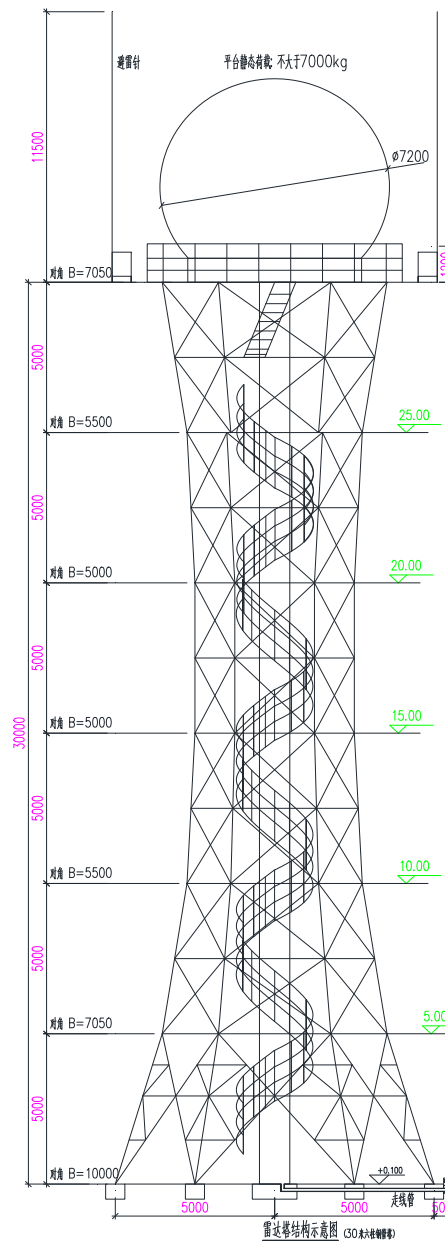
图 2-9 雷达塔结构示意图
