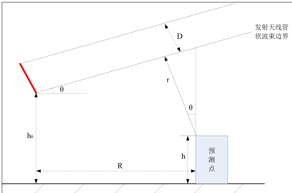
图 5-2 偏轴方向功率密度预测示意图
