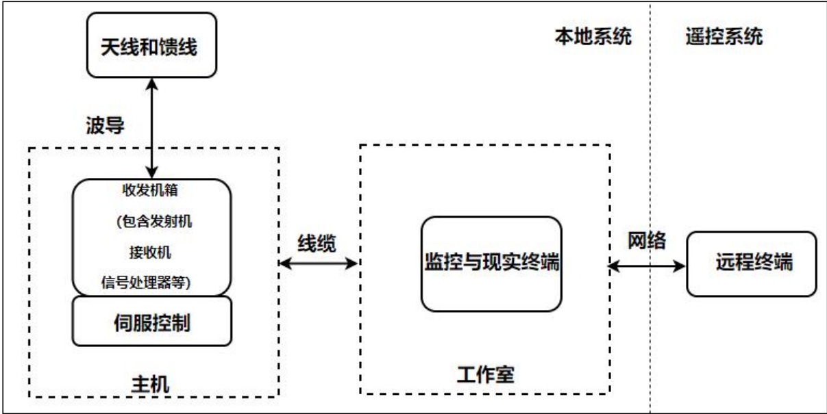
图 2-5 雷达系统组成示意图
