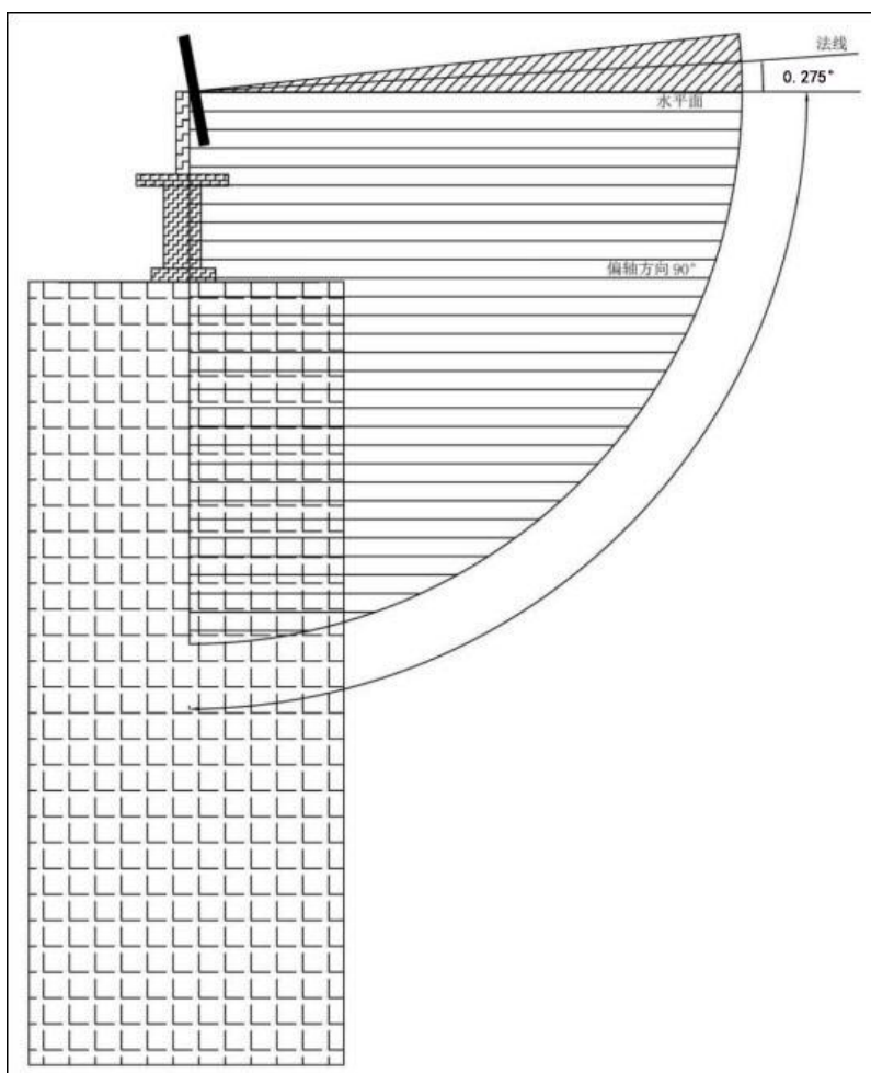
图 5-1 天线发射轴向、偏轴方向范围示意图
