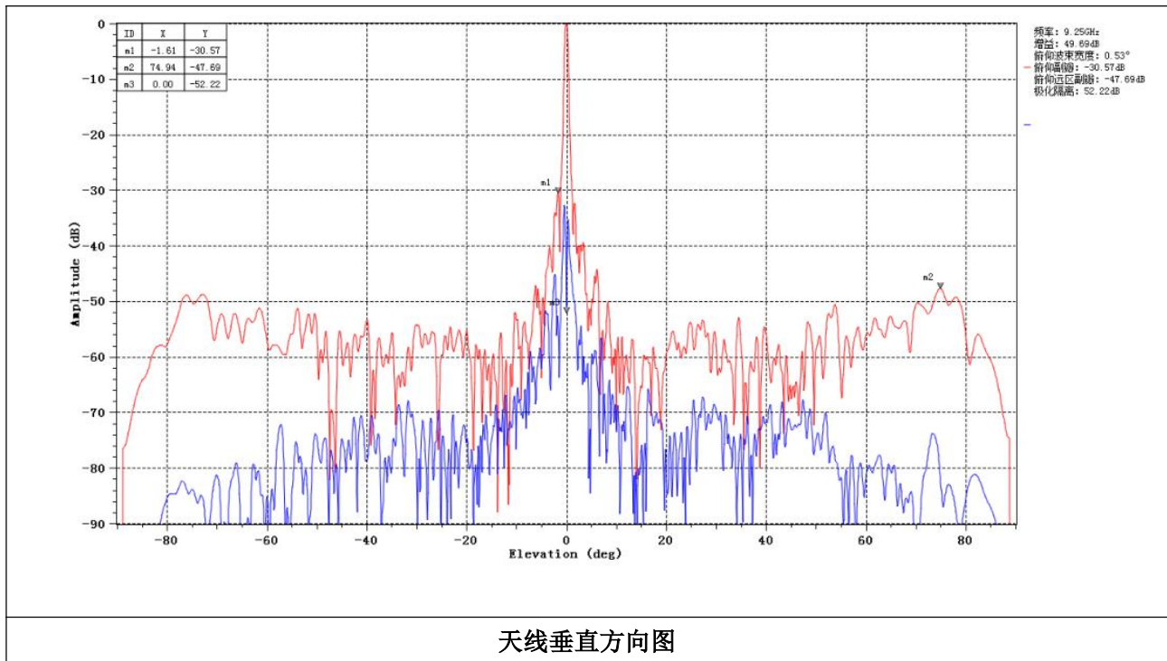
图 2-10 天线方向图
