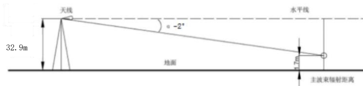
图 5-5 事故工况波束示意图
