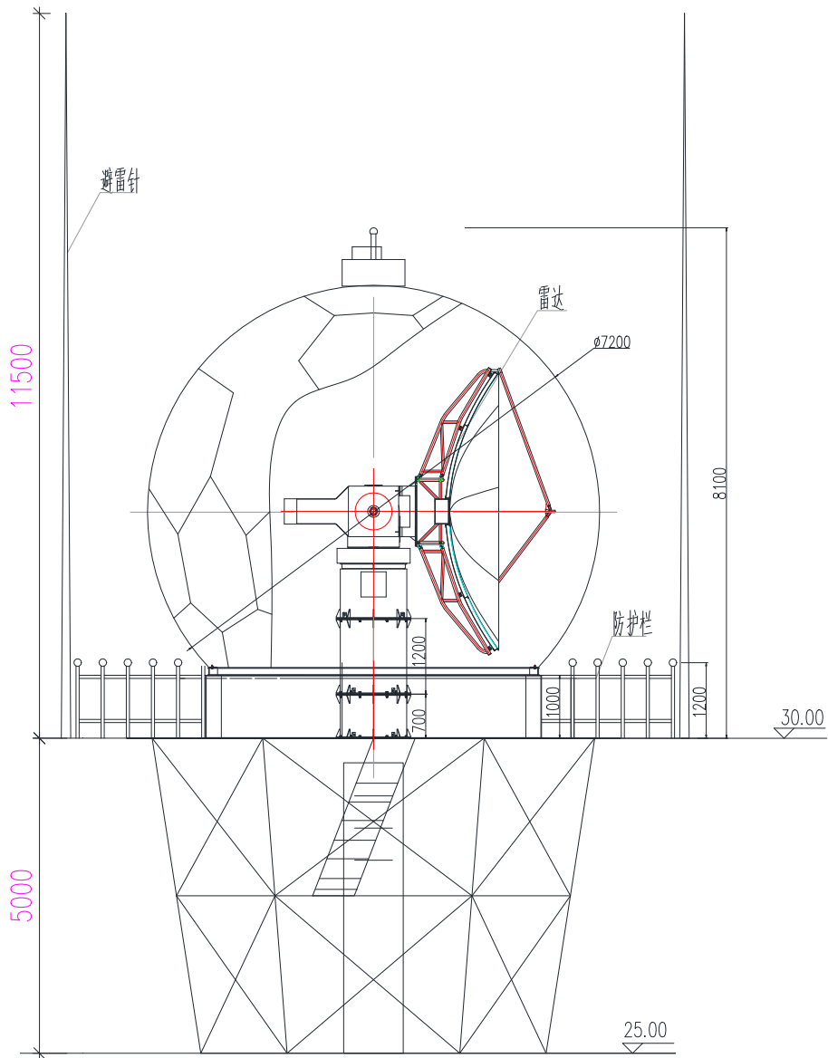
图 2-8 天线罩、天线底座结构示意图
