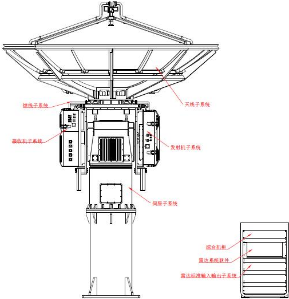
图 2-6 本项目雷达结构示意图
