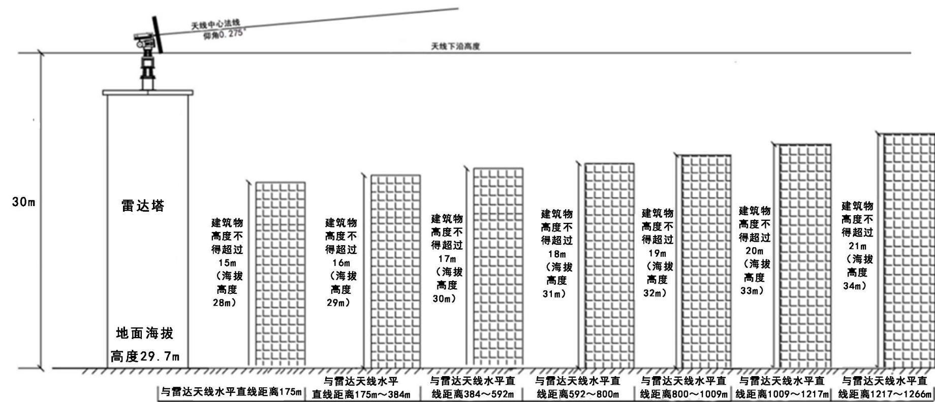
图 5-3 电磁环境控制范围及建筑物限高示意图（考虑波束仰角 0.275^\circ ）
